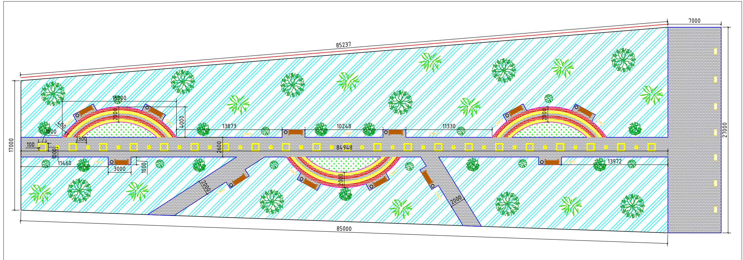
1. Светильник уличный
